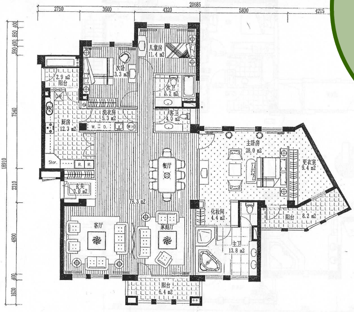
平面图 2#楼
